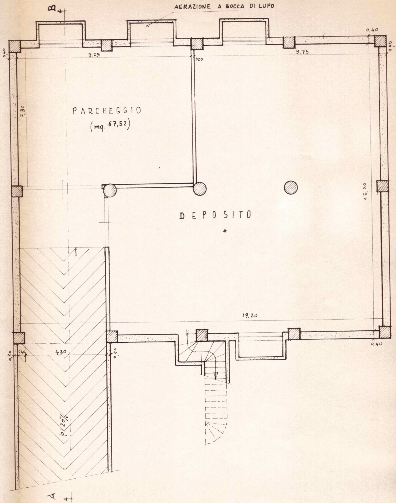
PIANTA PIANO INTERRATO
